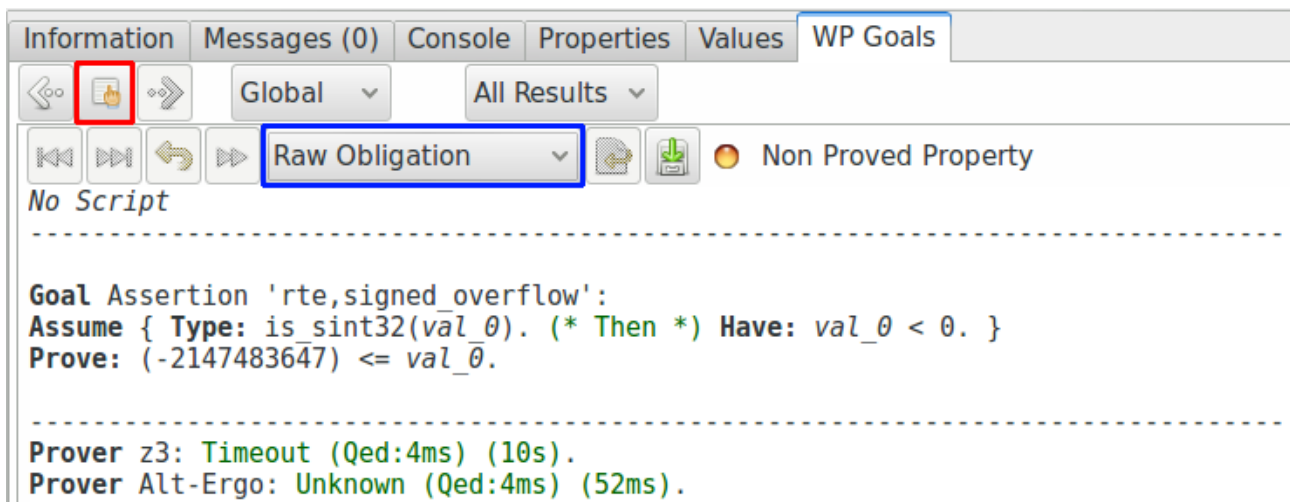
FIGURE 2.5. – Obligation de preuve associée à la vérification de débordement dans ‘abs’
