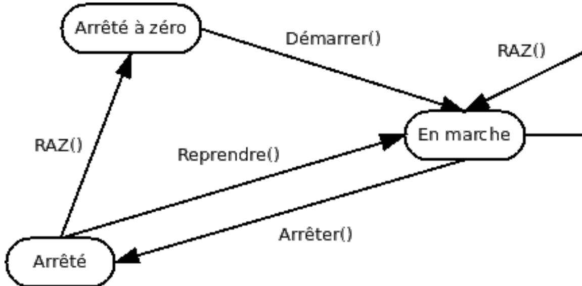
FIGURE 1.1. – Modélisation très abstraite d'un chronomètre
