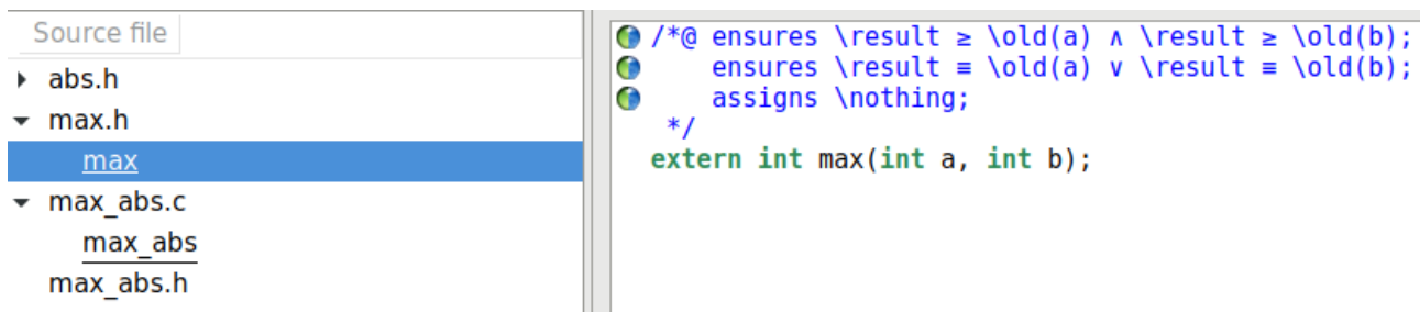
FIGURE 2.10. – Le contrat de ‘max’ est valide par hypothèse.
