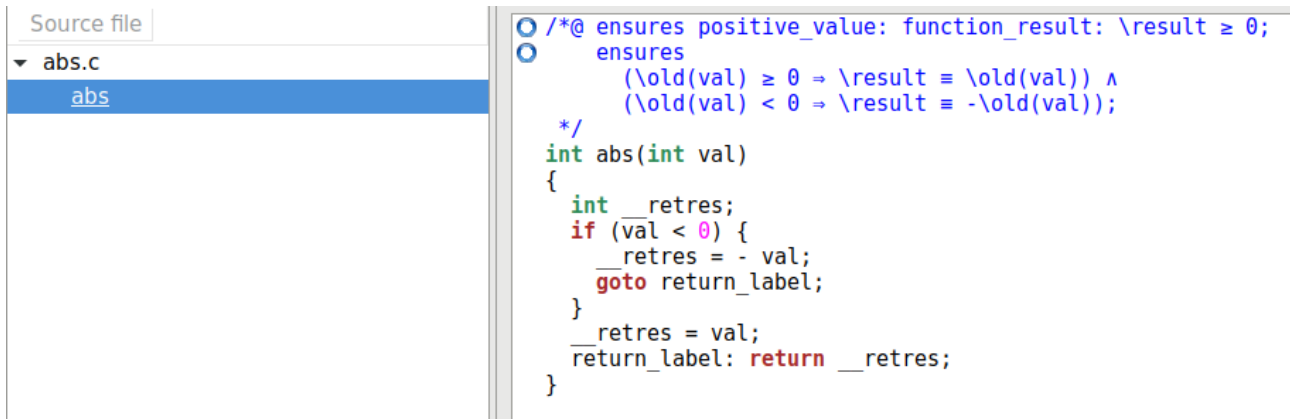
FIGURE 2.1. – Le volet latéral liste l’arbre des fichiers et des fonctions
