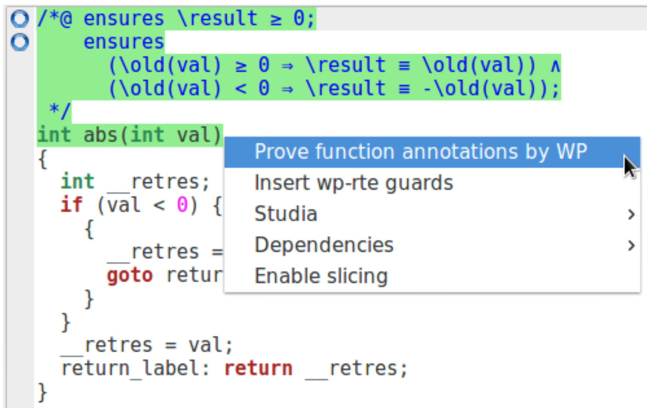
FIGURE 2.2. – Lancer la vérification de ‘abs’ avec WP
